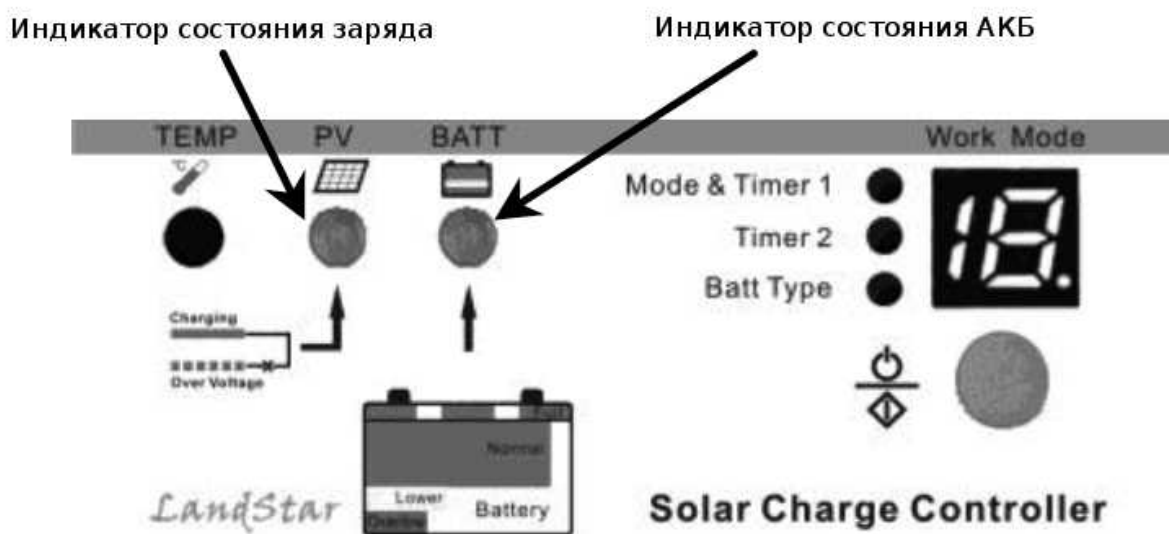
Рис. 4.2. Светодиодные индикаторы
